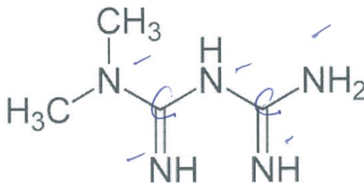
Metformin
