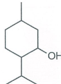
D – menthol
