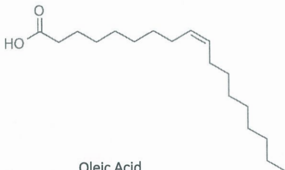
Oleic Acid
